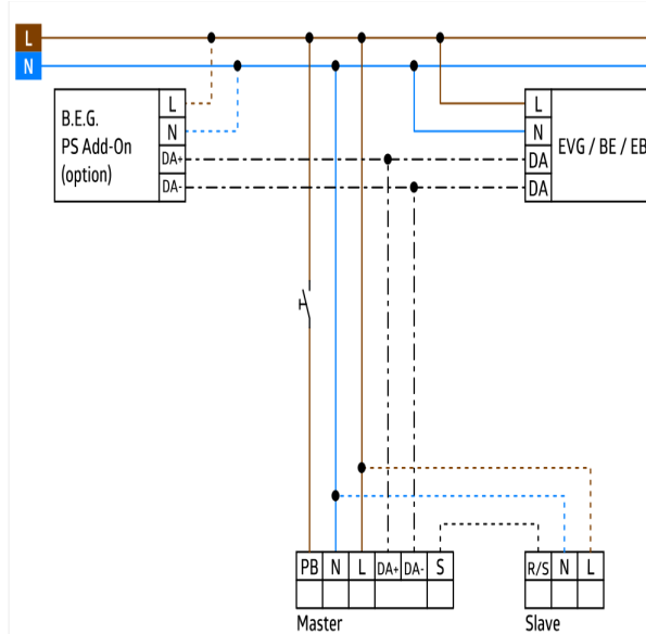
Schaltbild
