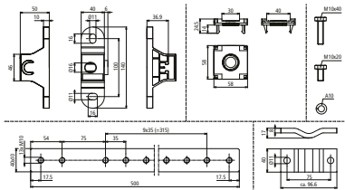
Maßbild PAS EX 1+9AP M10 V2A
