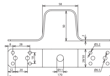
Maßbild UEBL L170 B11 B5.2 6.5 AL
