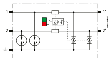
Prinzipschaltbild BCO CL2 BE 48
