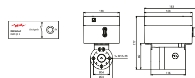
Maßbild DSRT QD II
