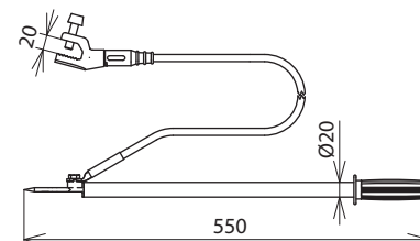
Maßbild EV TES 465 EK
