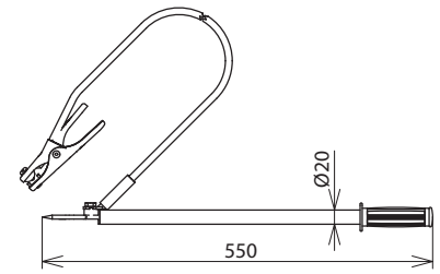
Maßbild EV TES 465 EZ
