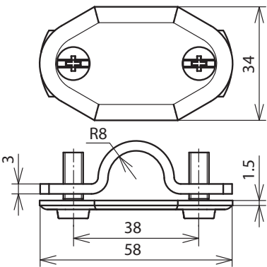
Maßbild NS 16 OZ AL
