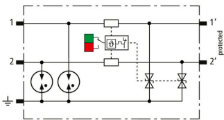
Prinzipschaltbild BCO CL2 BE 48
