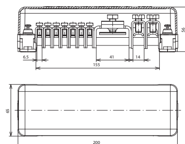
Maßbild PAS AH RK 7X25 2X8.10 1XFL40
