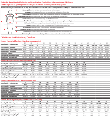
Maßbild APT OD YE 60
