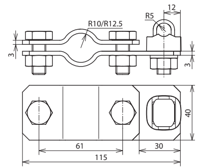
Maßbild AS TE 25 KSV 7.10 STTZN
