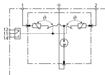
Prinzipschaltbild DR M 2P 255 SN1803FM
