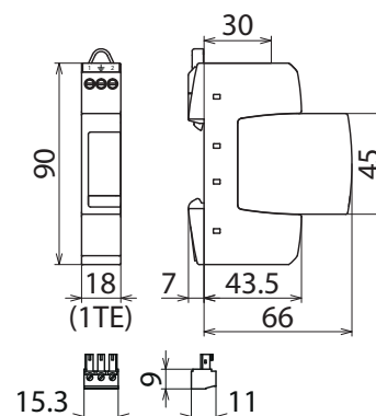
Maßbild DR M 2P 255 SN1803FM
