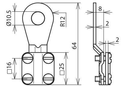
Maßbild EKSG 10 AQ6 16 CUGALZN
