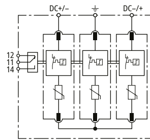
Prinzipschaltbild
