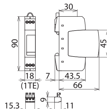
Maßbild DR M 2P 60 FM
