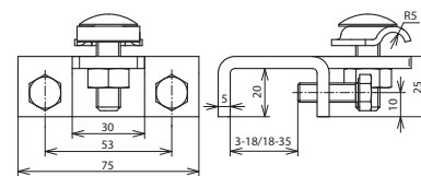
Maßbild AK 6.10 KB W KBF3 18 STTZN
