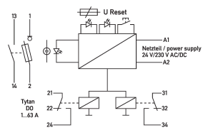
Anschlussschema
