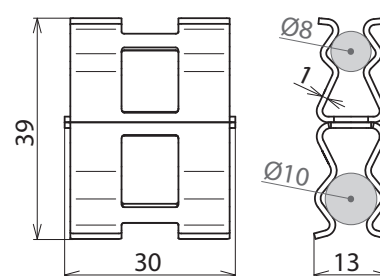
Maßbild DC BK 8 RD10 STBLANK
