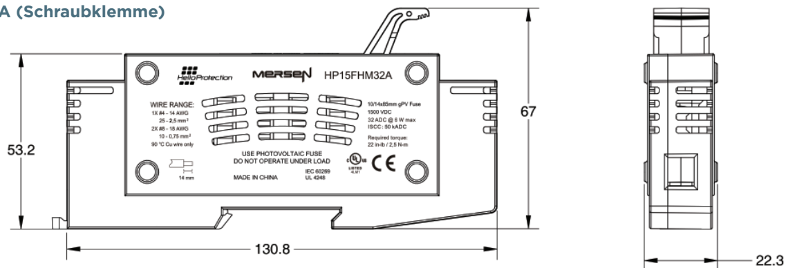
HP15FHM32A (Schraubklemme)
