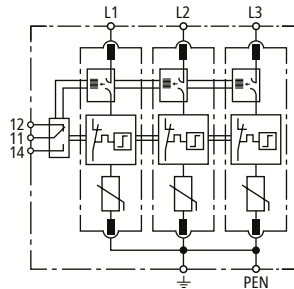
Prinzipschaltbild DG M TNC ACI 275 FM
