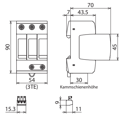
Maßbild DG M TNC ACI 275 FM
