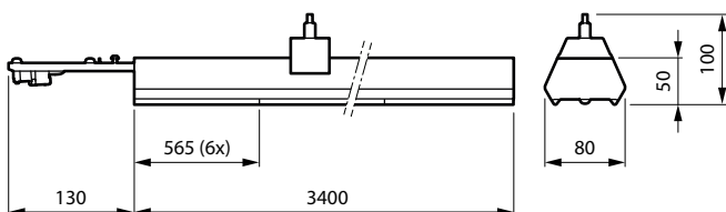
LL234X 90S/840 1x SIA NB 7x1.5
