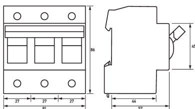
Maßzeichnung Gruppenansicht
