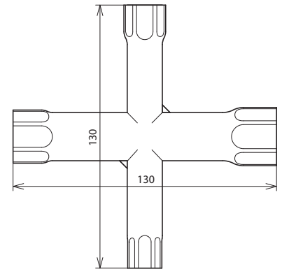
Maßbild KSS SW10 13 17 19 STGALZN
