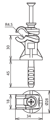
Maßbild LH DFI DQ 6.10 STTZN H30 GR
