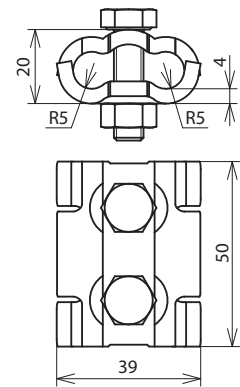
Maßbild PV 4.10 SKM8X30 STTZN
