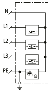
Prinzipschaltbild
