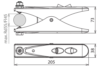
Maßbild
