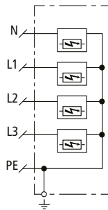
Prinzipialschaltbild
