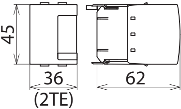
Maßbild DBH MOD 255
