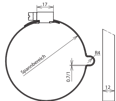
Maßbild LH 8 SB100.120 SCG GALCU
