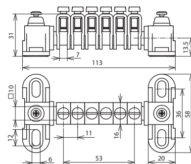
Maßbild PAS 6RK OH
