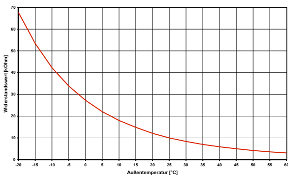
Abb. 7.2:Fühlerkennlinie NTC 10
