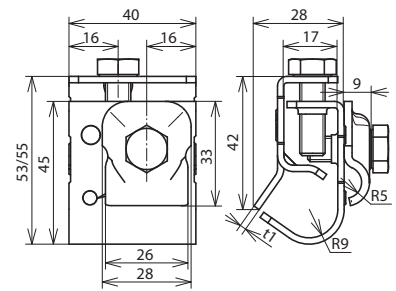
Maßbild DRK KB 6.10 W16.22 V2A
