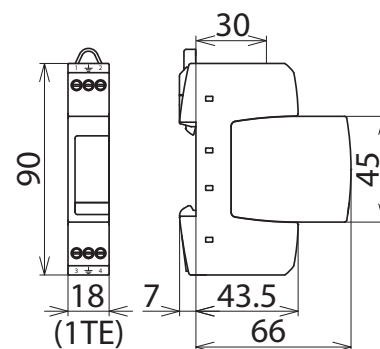
Maßbild DR M 2P 75
