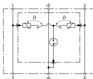
Prinzipschaltbild DR M 2P 75
