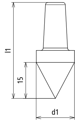
Maßbild SSP TE 25 TGTZN
