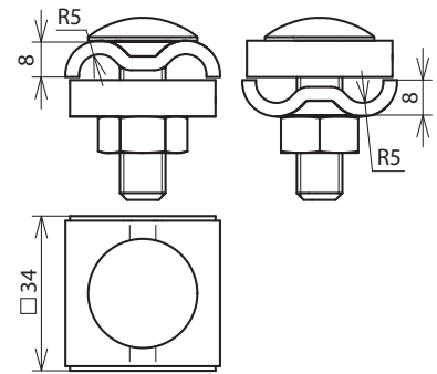
Maßbild UV 8.10 KTP V2A
