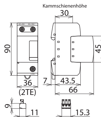
Maßbild DSE M 1 220 FM
