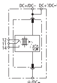
Prinzipialschaltbild DSE M 1 220 FM
