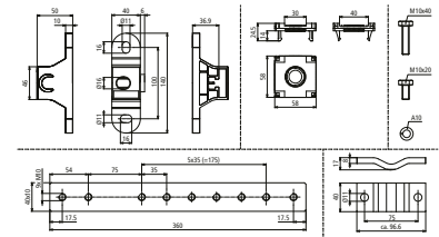
Maßbild
