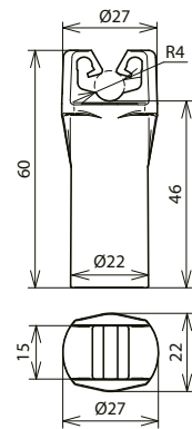
Maßbild DILH 8 SB10 K GR
