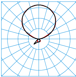
LuceoS S-U SMC PAW-IL 300-840 ETDI 03 (LEO1) TX369216 ■ C0 - C180 ■ C90 - C270 DIN 5040: E03 UTE: 0,08 D + 0,91 T CEN Flux Code: 53 86 96 8 100 49 82 98 92
