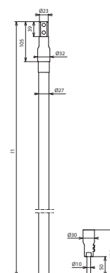
Maßbild HVI P RAV 90 27 L6M SW
