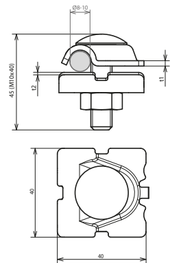
Maßbild MVK AR 8.10 FRM10X40 V4A
