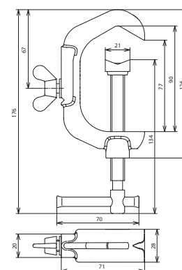
Maßbild EK 12.60 AQ6 16 TGTZN
