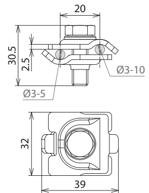
Maßbild MMVK 3.5 8.10 SKM8X30 V4A
