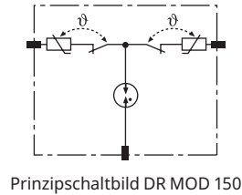
Prinzipialschaltbild DR MOD 150
