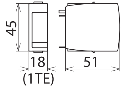
Maßbild DR MOD 150
