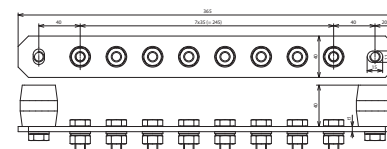
Maßbild PAS I 8AP M10 CU
