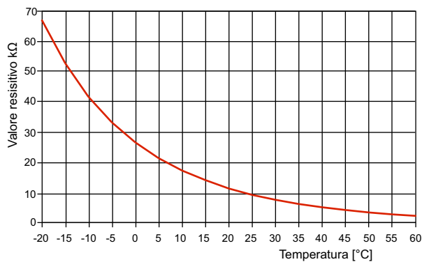
Abb. 3.3: Curva caratteristica della sonda NTC-10 per collegamento alla regolazione
