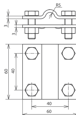
Maßbild KS 8.10 FL30 V4A
