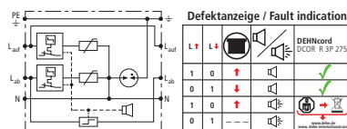
Prinzipschaltbild DCOR R 3P 275
