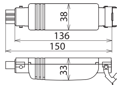
Maßbild DCOR R 3P 275
